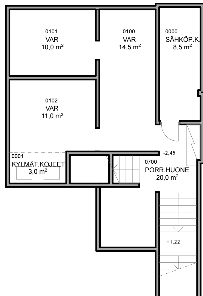
POHJAKUVA, KELLARI
